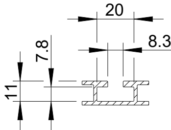
T-Nut/ T-slot
