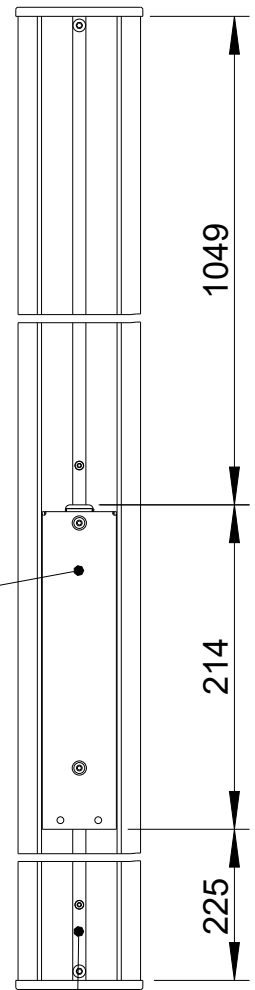
Rückansicht/ Rear view
