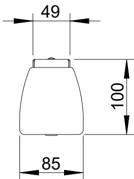
Draufsicht mit Abdeckung/ Top view with cover
