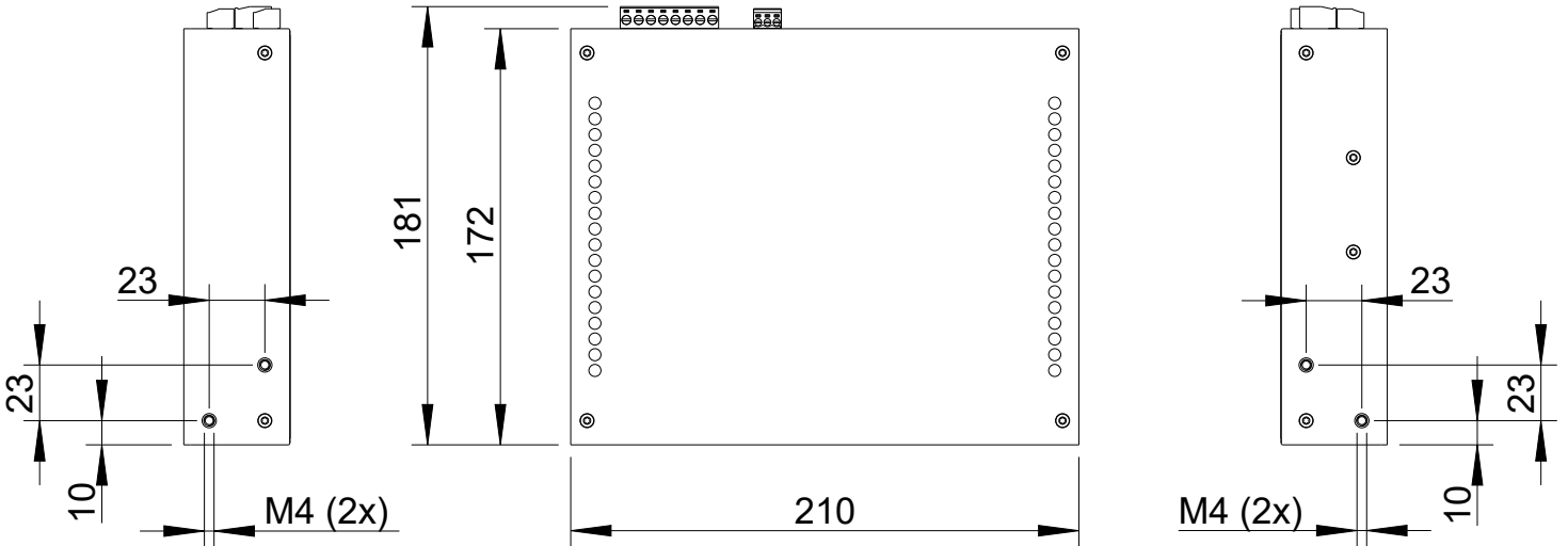
Seitenansicht rechts / Side view right
