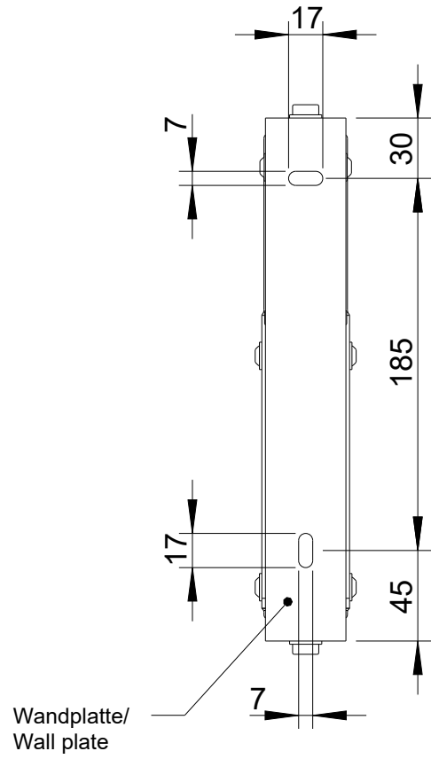
Rückansicht/ Rear view
