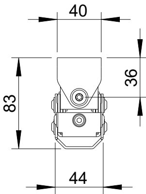
Draufsicht/ Top view
