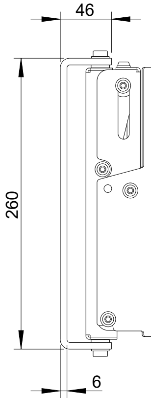
Seitenansicht/ Side view
