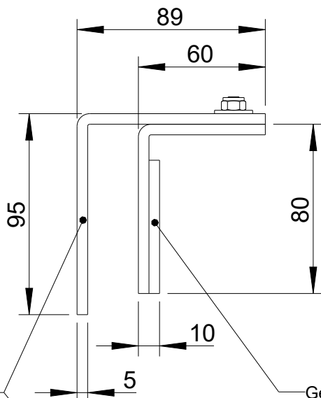
Seitenansicht/ Side view
