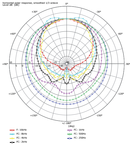
Bild 1: Polardiagramm horizontal
