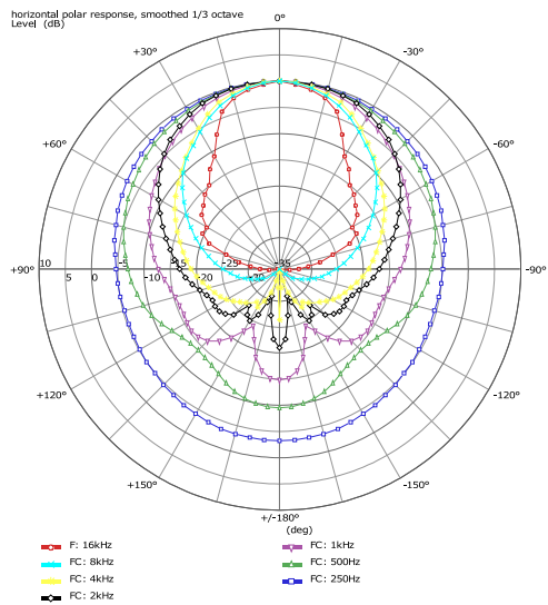
Abbildung 2: AT-201 60x40 Horizontal polar response
