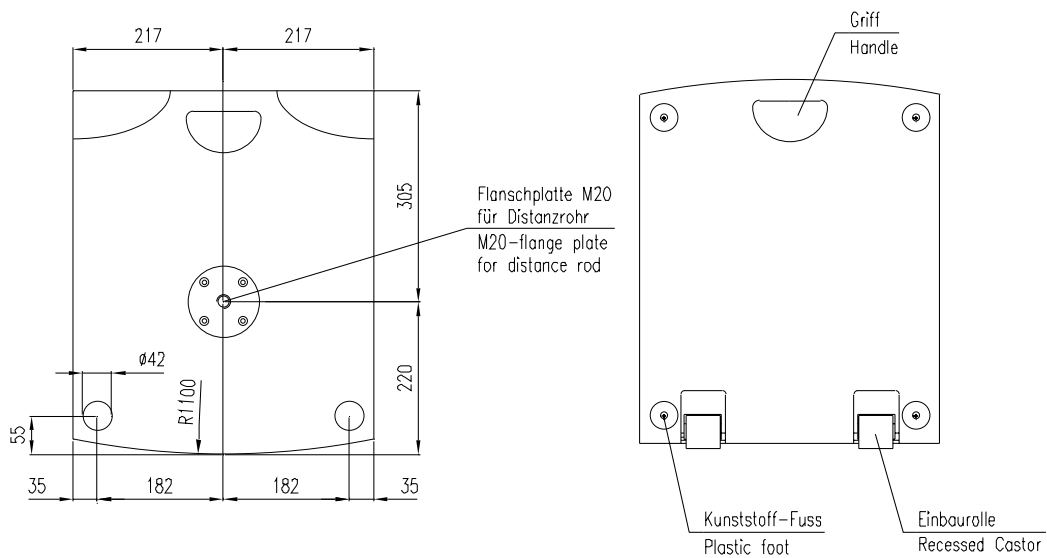
Bodensicht / Bottom view
