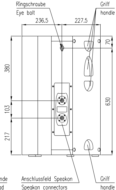
Rückansicht / Rear view
