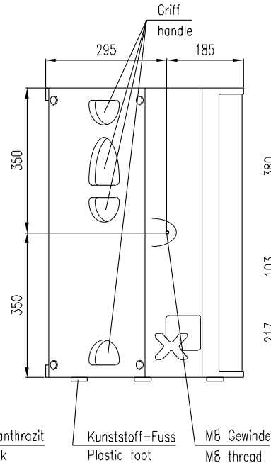
Seitenansicht / Side view
