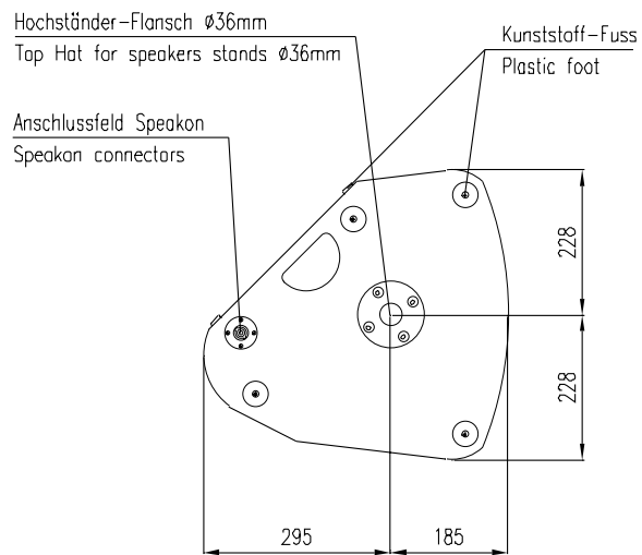
Ansicht von unten / Bottom view
